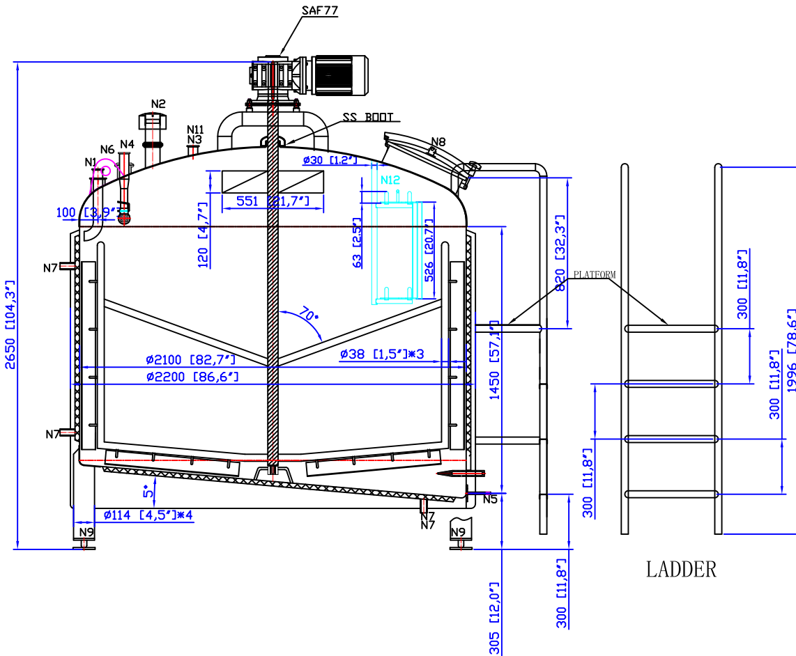
AGITATOR
